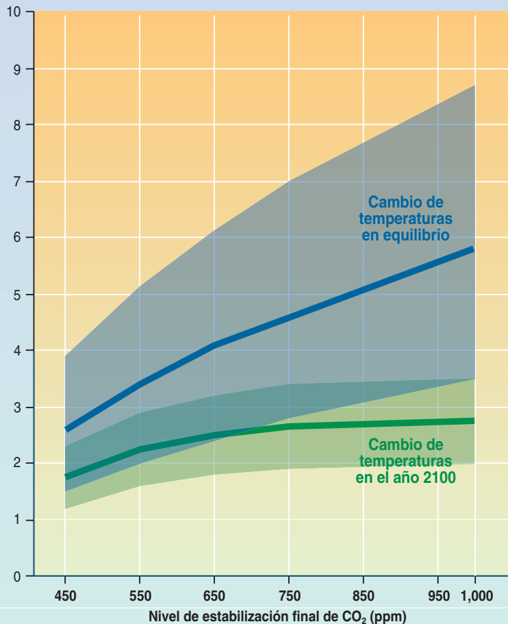
Figura RRP-7: Las concentraciones de CO 2 para la estabilización podrían disminuir el calentamiento, pero en un grado incierto.
