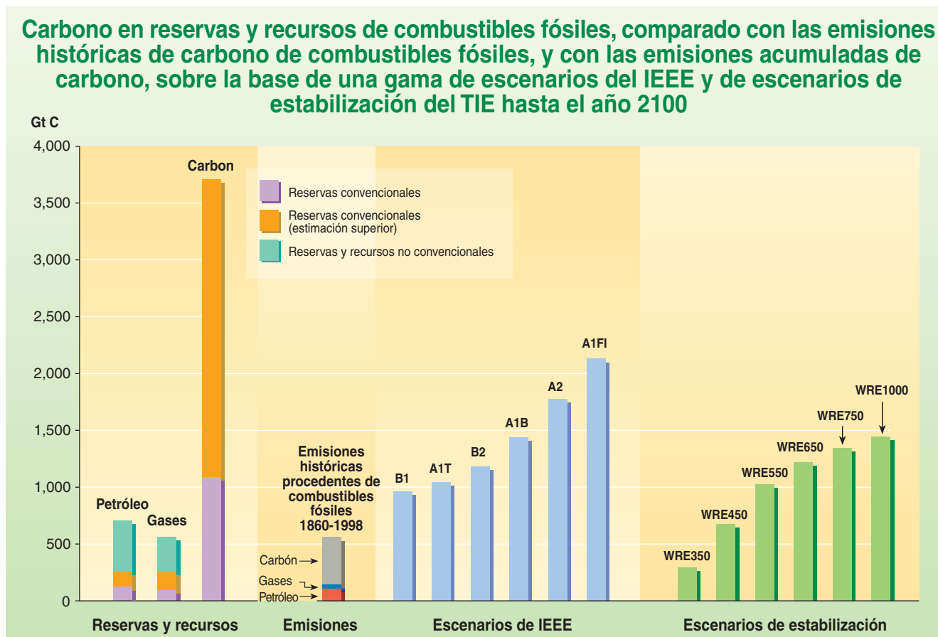
Figura 7-5: El carbono contenido en las reservas y recursos de petróleo, gas y carbón se compara con las emisiones históricas de carbono de combustibles fósiles durante el período 1860-1998, y con las emisiones acumuladas de carbono de una gama de escenarios del IEEE y escenarios de estabilización TIE hasta el año 2100. En las columnas de la izquierda se muestran los datos para las reservas y recursos actuales. El gas y el petróleo no convencionales incluyen arenas asfálticas, esquistos de petróleo, otros aceites pesados, metano en lechos de carbón, gas geopresurizado, gas en acuíferos, etc. No se muestran los hidratos de gas (clatratos) que ascienden a una cantidad estimada de 2.000 Gt C. Las columnas del escenario muestran los escenarios de referencia del IEEE y los escenarios que llevan a una estabilización de las concentraciones de CO 2 a una gama de niveles. Conviene observar que si para el año 2100 las emisiones acumuladas asociadas con los escenarios del IEEE son iguales o menores a las de los escenarios de estabilización, ello no implica que estos escenarios lleven igualmente a la estabilización.
