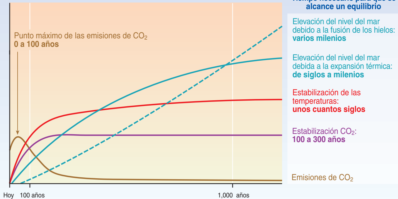
Figura RRP-5: Después de reducirse las emisiones de CO 2 y de que se establezcan las concentraciones atmosféricas, la temperatura de la atmósfera en la superficie terrestre ha de continuar incrementándose lentamente durante un siglo o más.
