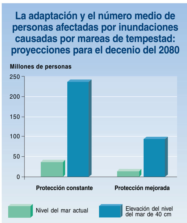
Figura 3–6: La adaptación y el número medio de personas afectadas por inundaciones causadas por mareas de tempestad en las costas: proyecciones para el decenio del 2080. Las dos barras de la izquierda muestran el número de personas afectadas por inundaciones debidas a mareas de tempestad costeras en el año 2080 respecto al nivel del mar actual y para una elevación del nivel del mar de ~40 cm, suponiendo que la protección costera no cambia a partir de ahora y que haya un aumento demográfico moderado. Las dos barras a la derecha muestran lo mismo, pero suponiendo que la protección costera se mejora en proporción al crecimiento del PIB.
