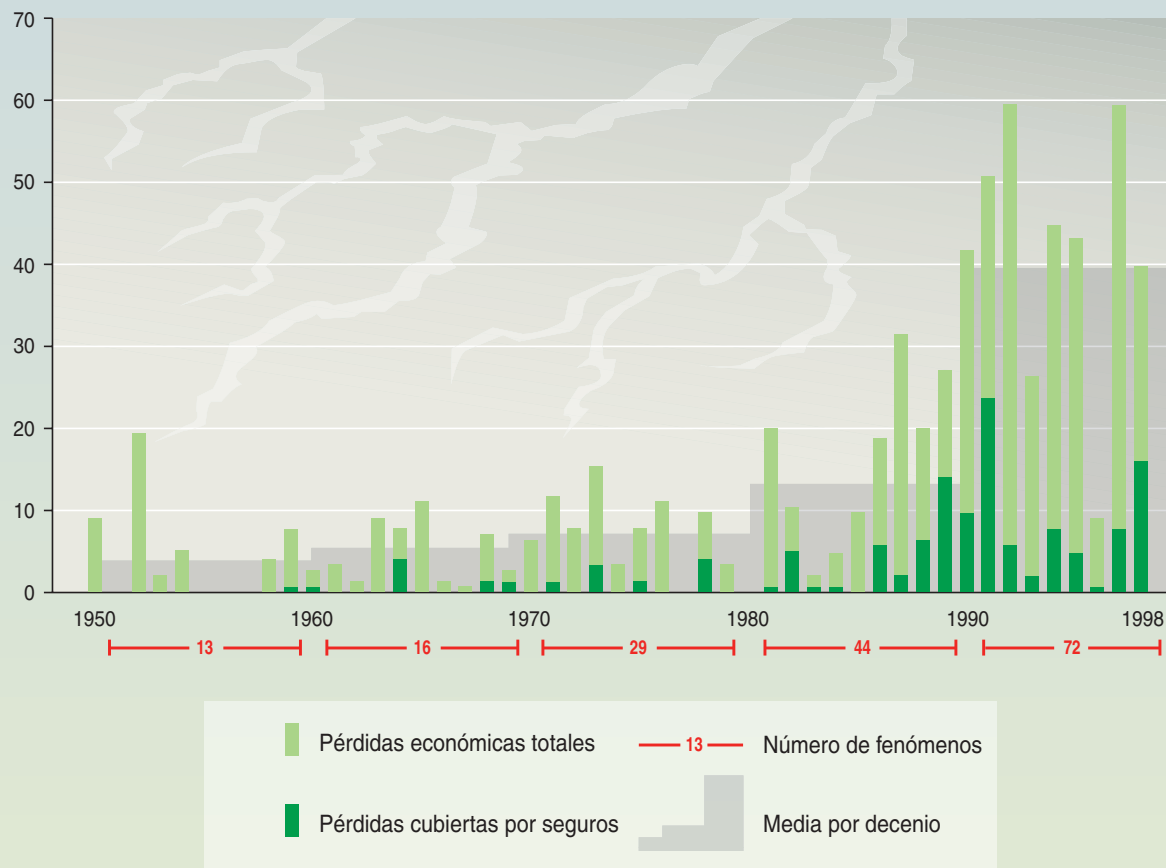
Figura 2-7: Las pérdidas económicas ocasionadas por fenómenos meteorológicos catastróficos se han multiplicado mundialmente por diez (con ajustes para la inflación) entre los decenios de 1950 y de 1990, mucho más rápidamente de lo que se pudiera explicar con la simple inflación.
