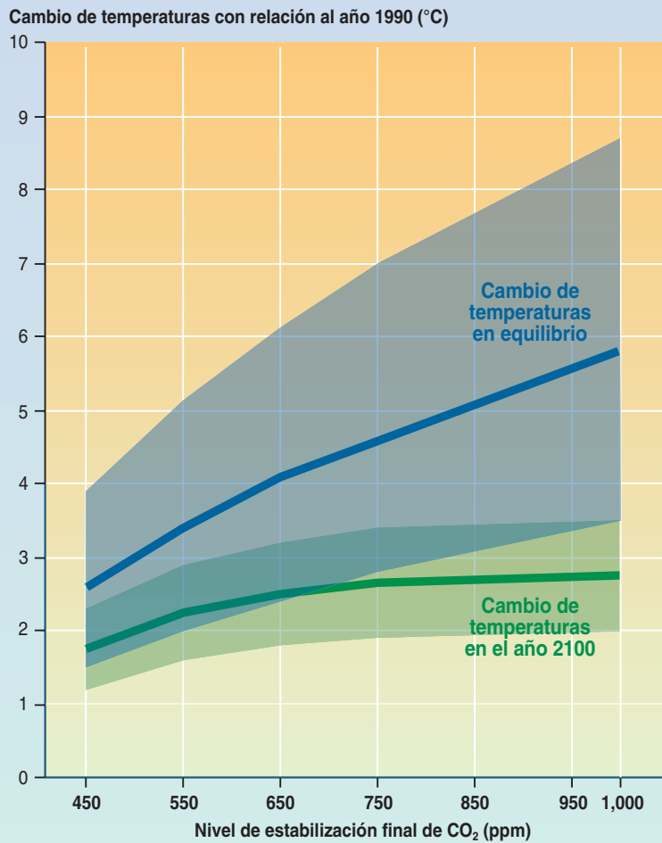
Figura 6-2: Los cambios de temperatura con relación al 1990 en: a) el año 2100, y b) en equilibrio, se estiman utilizando una simulación climática sencilla para los perfiles WRE, como en la Figura 6-1. Las estimaciones mínimas y máximas para cada nivel de estabilización suponen una sensibilidad climática de 1,7 y 4,2°C, respectivamente. La línea central es una media de las estimaciones máximas y mínimas.
