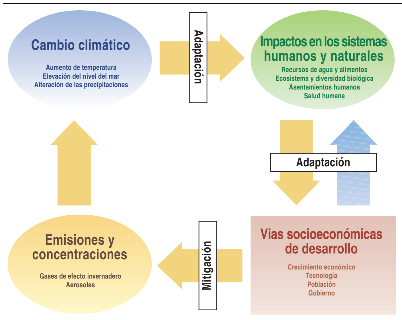
Figura RRP-1: Cambio climático—un marco integrado. Representación esquemática y simplificada de un marco de evaluación integrado para la consideración de los cambios climáticos antropogénicos. Las flechas amarillas muestran el ciclo de causa a efecto entre los cuatro cuadrantes mostrados en la figura, y la flecha azul indica la respuesta de la sociedad ante los impactos del cambio climático. Véase una descripción más detallada de este marco, al pie de la Figura 1-1.
