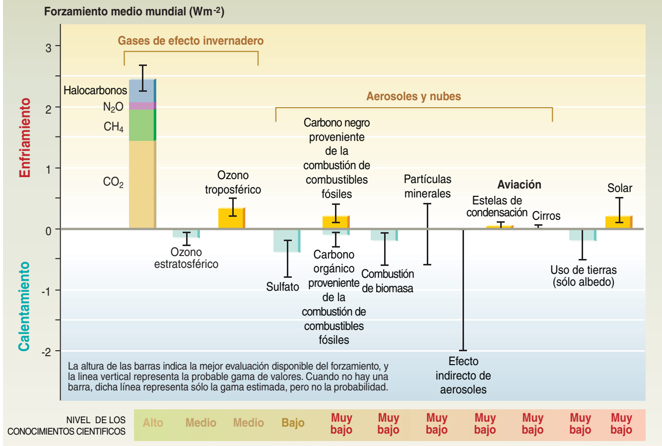
Figura 2-2: La influencia de los factores externos sobre el clima puede compararse en términos generales utilizando el concepto de los forzamientos radiativos. Dichos forzamientos radiativos surgen de los cambios en la composición atmosférica, la alteración de la reflectancia de la superficie terrestre, debida a cambios en el uso de las tierras, y la variación de la producción del sol. Con la excepción de la variación solar, hay alguna forma de actividad humana asociadas con cada uno de estos fenómenos. Las barras rectangulares representan las estimaciones de estos forzamientos, algunos de los cuales producen calentamiento y otros, enfriamiento. No se muestran los forzamientos debidos a fenómenos volcánicos, que causan forzamientos negativos que sólo duran unos años. El efecto indirecto de los aerosoles que se indica son los efectos sobre el tamaño y el número de pequeñas gotitas en las nubes. Tampoco se muestra un segundo efecto indirecto de los aerosoles sobre las nubes, concretamente, su efecto sobre el tiempo de vida de la nube, lo que también produciría un forzamiento negativo. Los efectos de la aviación sobre los gases de efecto invernadero se incluyen en cada una de las barras. La línea vertical que se cruza las barras rectangulares indica una gama de estimaciones, que se guían por el abanico de los valores publicados de los forzamientos y por nuestros conocimientos actuales de los aspectos físicos del fenómeno. Algunos de estos forzamientos presentan un mayor grado de certeza que otros. Una línea vertical sin una barra rectangular denota un forzamiento para el que no se puede dar una mejor estimación debido al gran número de incertidumbres. Tal como se ha indicado, el nivel general de nuestros conocimientos científicos sobre cada uno de los forzamientos varía considerablemente. Algunos de los agentes de forzamiento radiativo (el CO 2 , por ejemplo) se encuentran muy mezclados por todo el planeta, desestabilizando el equilibrio mundial del calor. Otros (por ejemplo, los aerosoles) representan perturbaciones que son más poderosas en una regiones que en otras, ya que están distribuidas de forma irregular. Los forzamientos radiativos continúan siendo una herramienta muy útil para estimar, en primer lugar, los impactos relativos del clima, como la respuesta de la temperatura media relativa en la superficie de la Tierra debida a perturbaciones inducidas radiativamente, pero estas estimaciones de forzamientos medios relativos no son necesariamente indicadores de los aspectos detallados de posibles respuestas climáticas (por ejemplo, los cambios climáticos regionales).
