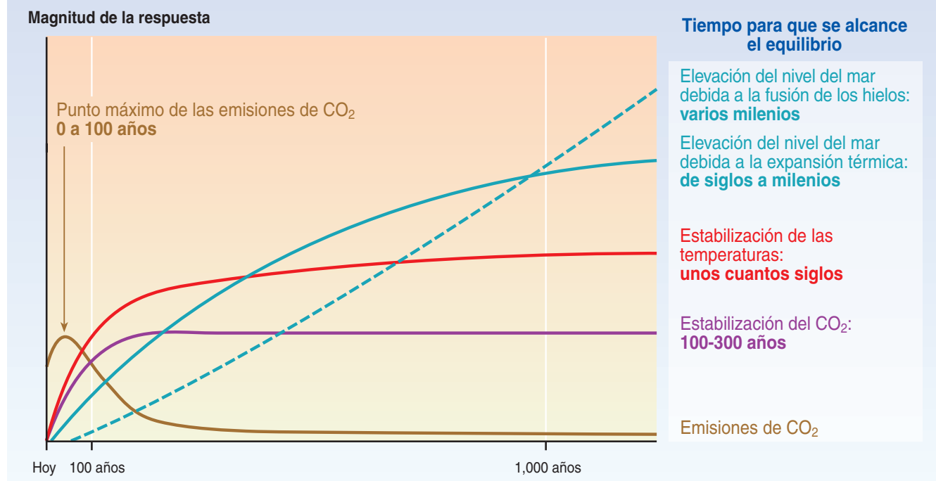
Figura 5-2: Después que se reduzcan las emisiones de CO 2 y que se estabilicen las concentraciones atmosféricas, la temperatura de la atmósfera en la superficie del planeta ha de continuar incrementándose en unas cuantas décimas partes de un grado C por siglo durante un siglo o más. La expansión térmica de los océanos ha de continuar incluso mucho después de haberse reducido las emisiones de CO 2 , y la fusión de las capas de hielo continuará contribuyendo durante muchos siglos a la elevación del nivel del mar. Esta figura es una ilustración genérica de la estabilización a cualquier nivel entre 450 y 1.000 ppm y, por lo tanto, no incluye unidades en el eje de respuestas. Las respuestas a las trayectorias de estabilización en esta serie muestran unos períodos similares, pero los impactos son progresivamente más acuciantes cuando existen mayores concentraciones de CO 2 .
