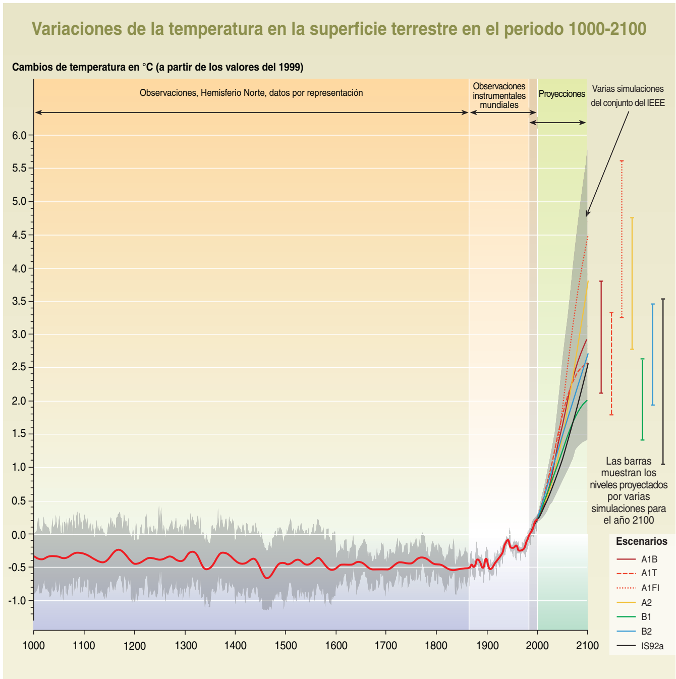
Figura RRP-10b: Se muestran las variaciones en la temperatura media de la superficie en el Hemisferio Norte durante el período 1000–1860 (no se dispone de los datos correspondientes para el Hemisferio Sur) extraídos a partir de datos por representación (anillos de los árboles, corales, testigos de hielo y registros históricos). La línea muestra una media en 50 años, el área gris, el límite de confianza del 95 por ciento en los datos anuales. Para el período 1860–2000 se muestran las observaciones de variaciones anuales y mundiales de la temperatura media de la superficie obtenidas del registro instrumental. La línea muestra la media por decenios. Para el período 2000–2100, se muestran las proyecciones de la temperatura media mundial de la superficie para los seis escenarios ilustrativos del IEEE y los del IS92a, estimadas mediante una simulación con sensibilidad climática media. El área gris marcada 'Varias simulaciones del conjunto del IEEE' muestra la gama de resultados de los 35 escenarios del IEEE además de aquellos obtenidos de una gama de simulaciones con diferentes sensibilidades climáticas. La escala de temperaturas se determina a partir del valor para 1990; la escala es diferente de la utilizada en la Figura RRP-2.
