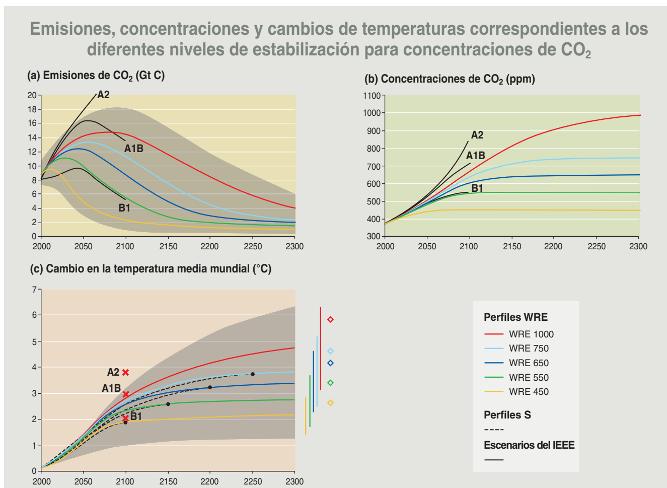
Figura RRP-6: La estabilización de las concentraciones de \text{CO}_2 requeriría una reducción importante de las emisiones por debajo de los niveles actuales, y frenaría la velocidad del calentamiento.
