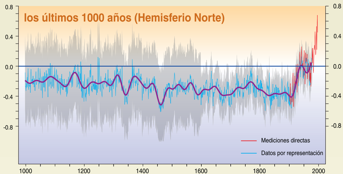
Figura 2-3: La temperatura de la superficie terrestre se ha incrementado en unos 0,6°C por encima del récord de mediciones directas de la temperatura (1860-2000, panel superior), aumento sin precedentes, al menos a juzgar por los datos de temperaturas obtenidos por representación en el Hemisferio Norte durante el último milenio (panel inferior).
